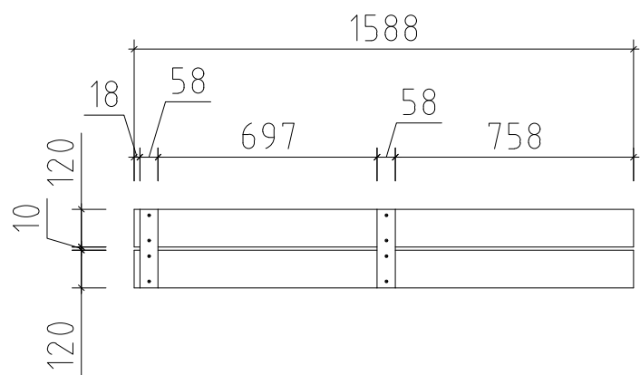
DACHBLENDEN 1a - PARAPET 1a
