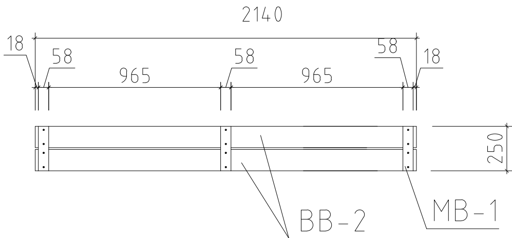
DACHBLENDEN 2 - PARAPET 2
