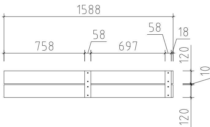
DACHBLENDEN 1b - PARAPET 1b
