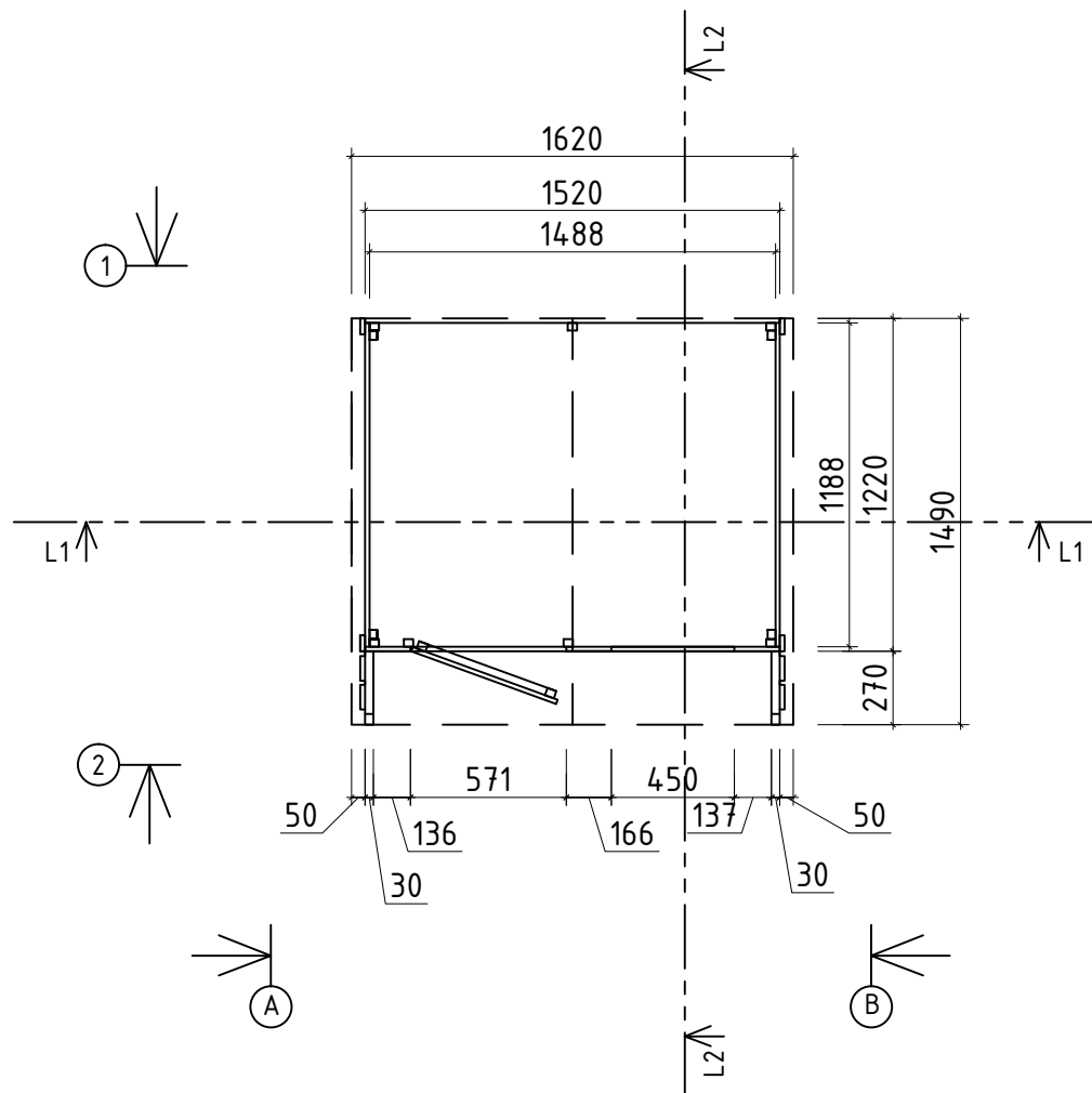
Alustaladeplaan / Lagerhölzplan / Foundation beams
